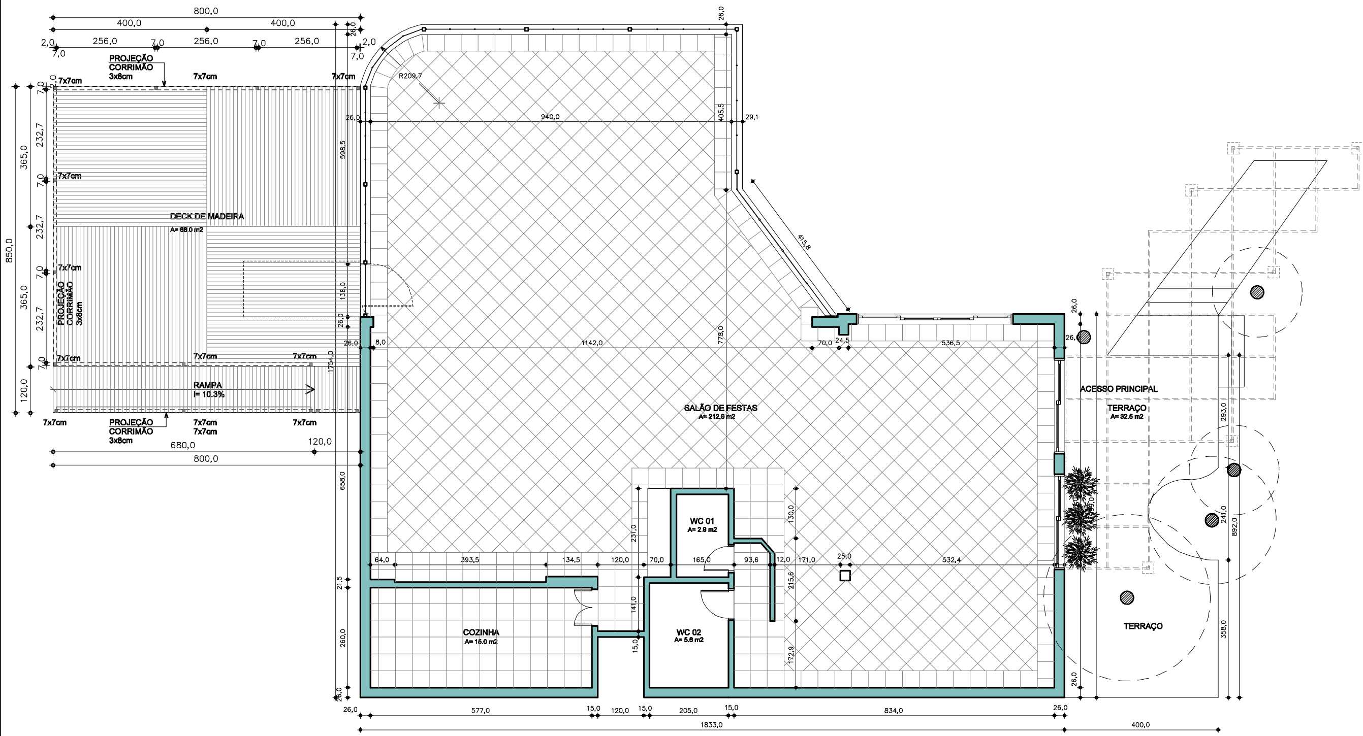
PLANTA BAIXA SALÃO IPANEMA ESC. 1/100
